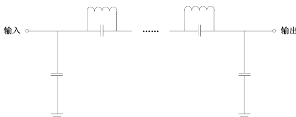
YLBP-2450-3150-B4产品原理图
