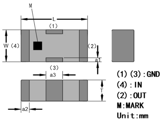
产品外形
