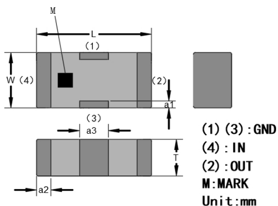
产品外形
