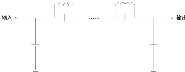
YLBP-3250-3950-B4产品原理图
