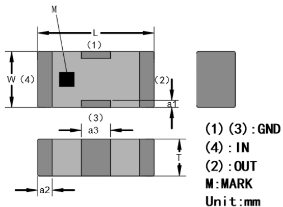
产品外形
