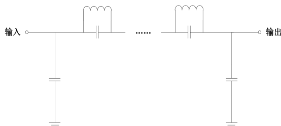
YLLP-2900-E4产品原理图
