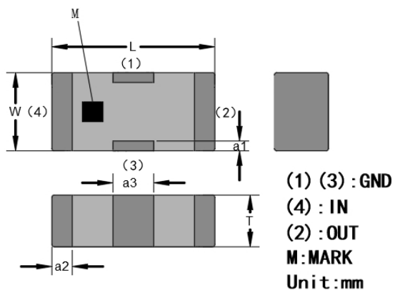
产品外形
