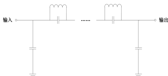
YLLP-1800-E4产品原理图
