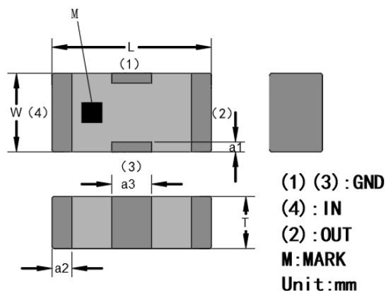
产品外形
