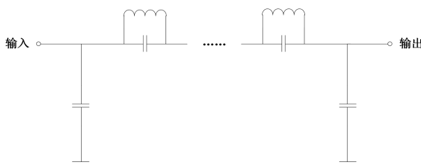
YLBP-3450-4150-B4产品原理图
