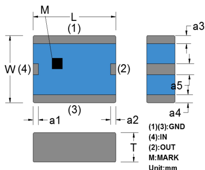
产品外形
